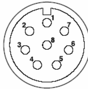
Vista del conector Lemo1-B de 8 terminales
