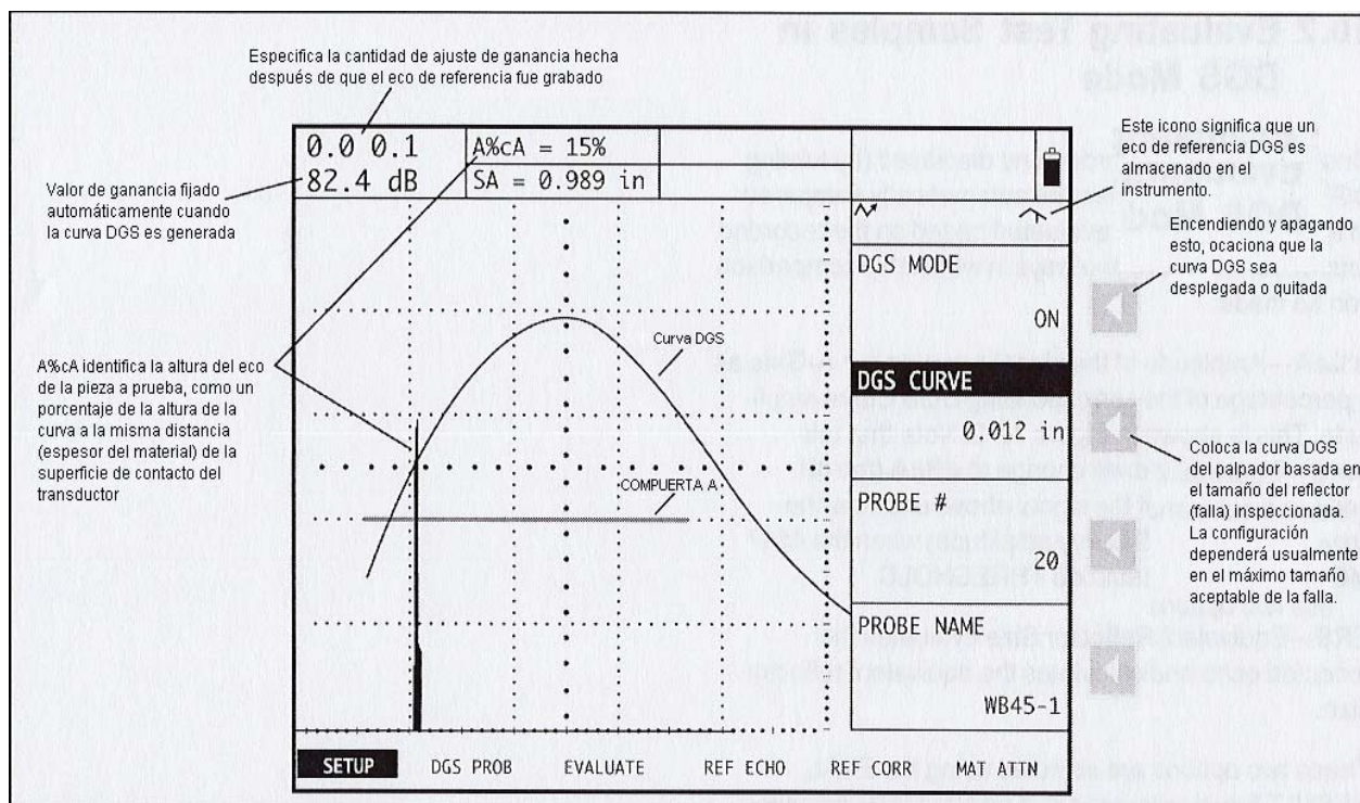
FIGURA 10-2—Curva DGS
