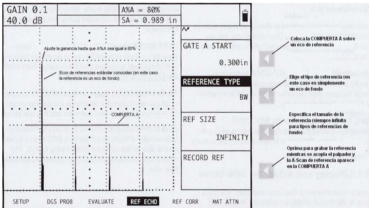
FIGURA 10-1—Grabando un punto de referencia DGS desde el cuál una curva DGS será generada
